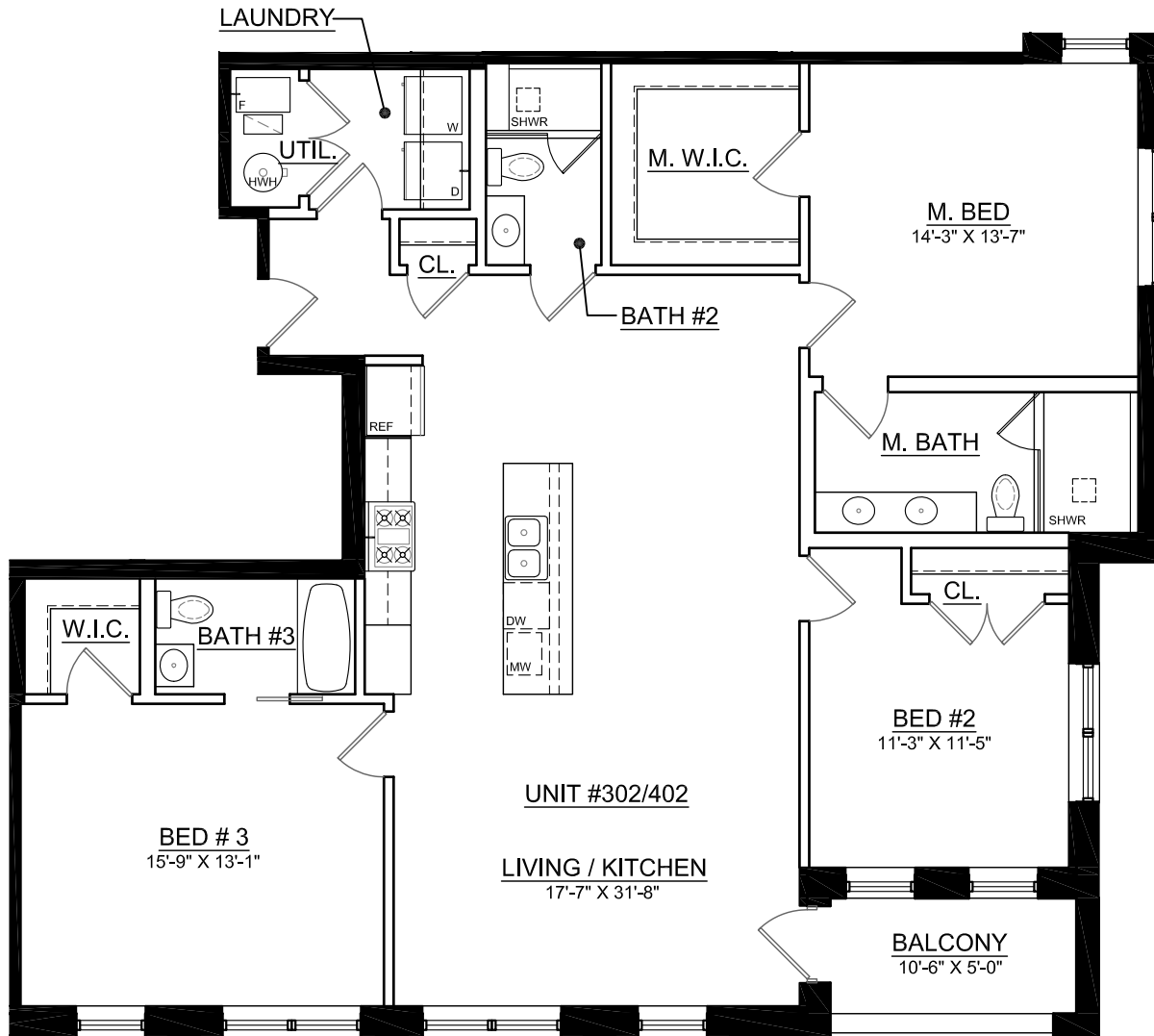
UNIT 302 / 402 SCALE: 1/8" = 1'-0"
