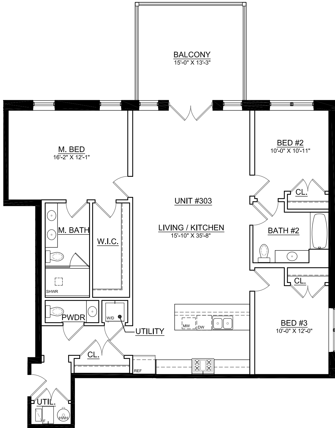
UNIT 303 SCALE: 1/8" = 1'-0"
