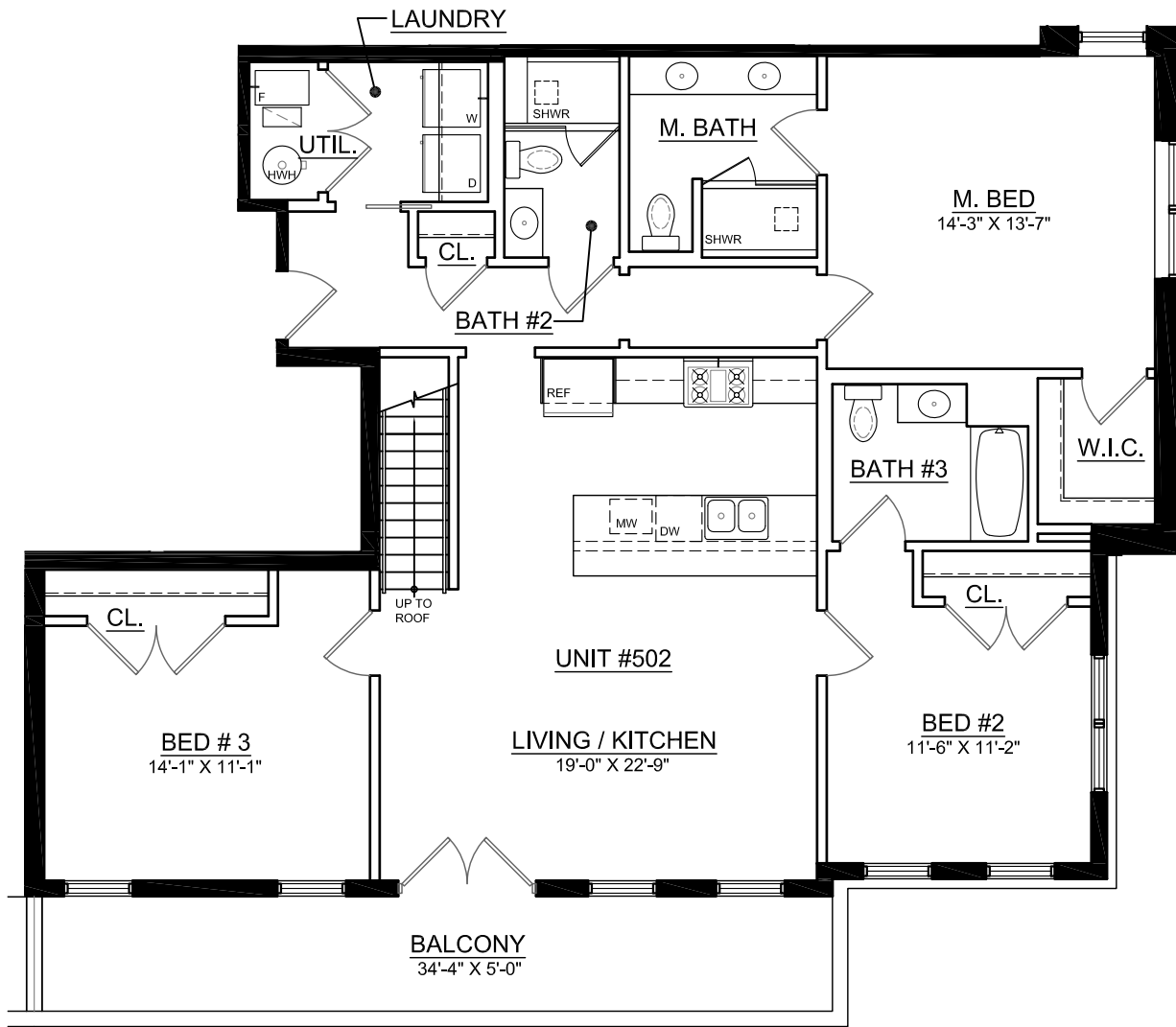
UNIT 502 SCALE: 1/8" = 1'-0"
