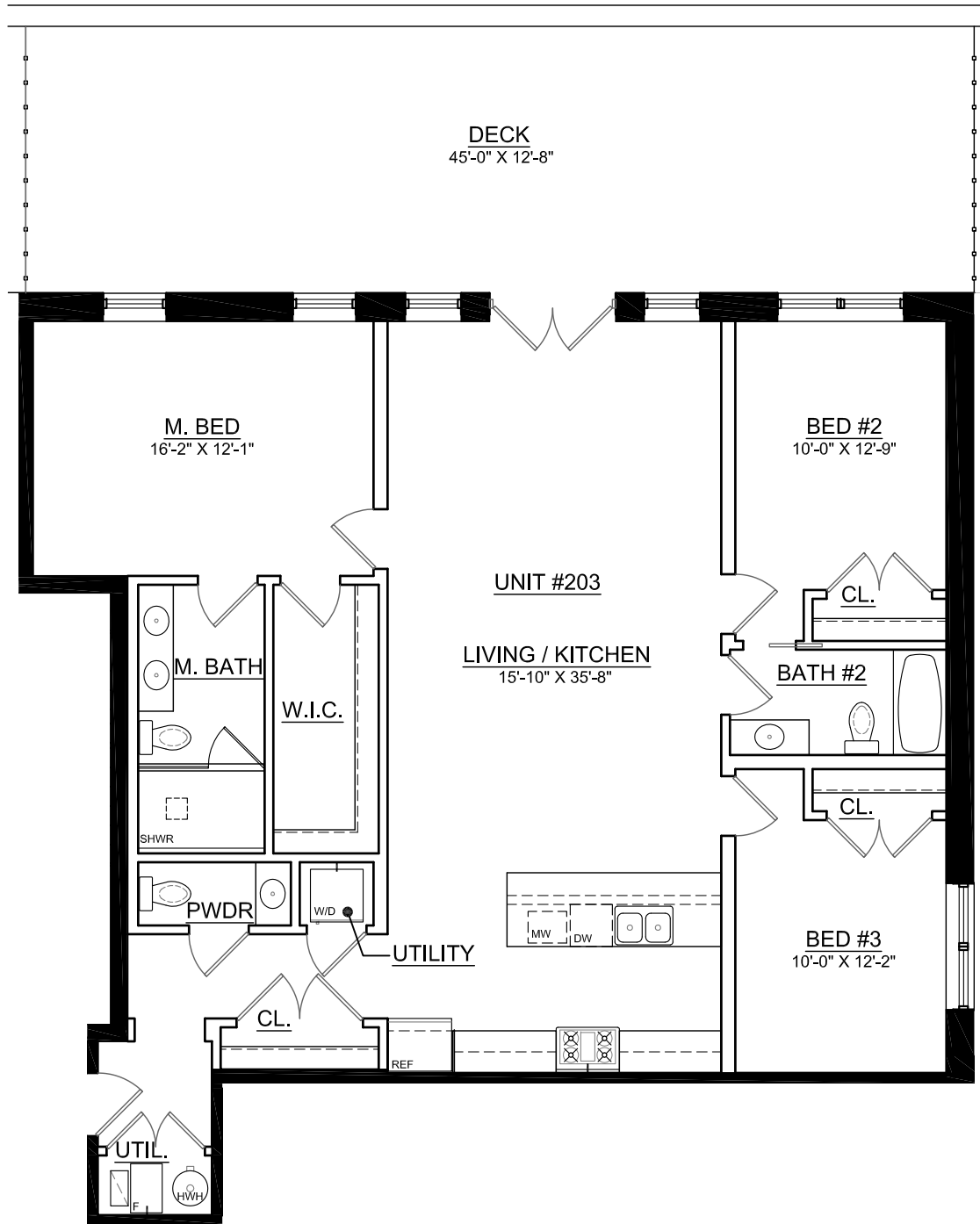
UNIT 203 SCALE: 1/8" = 1'-0"
