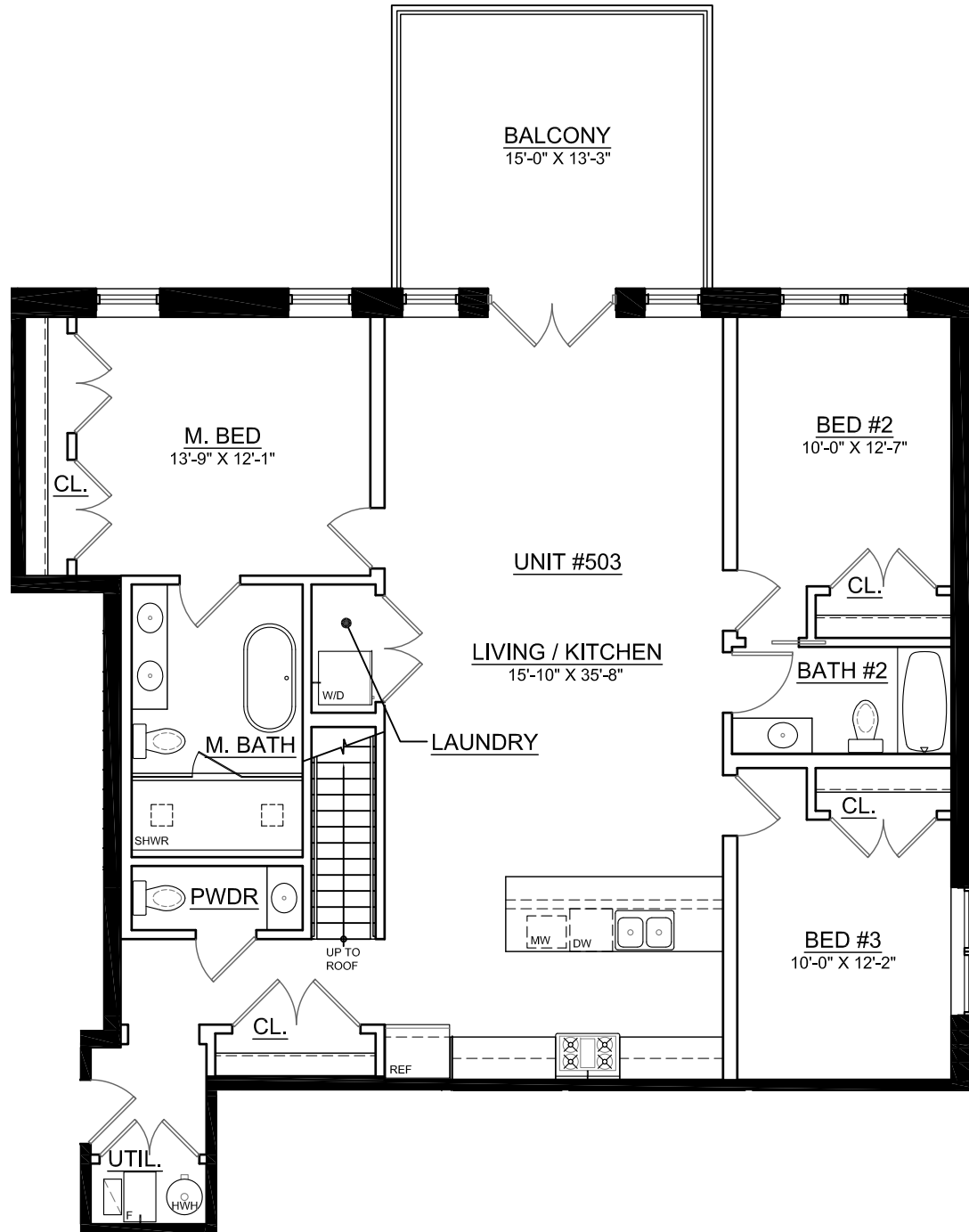
UNIT 503 SCALE: 1/8" = 1'-0"
