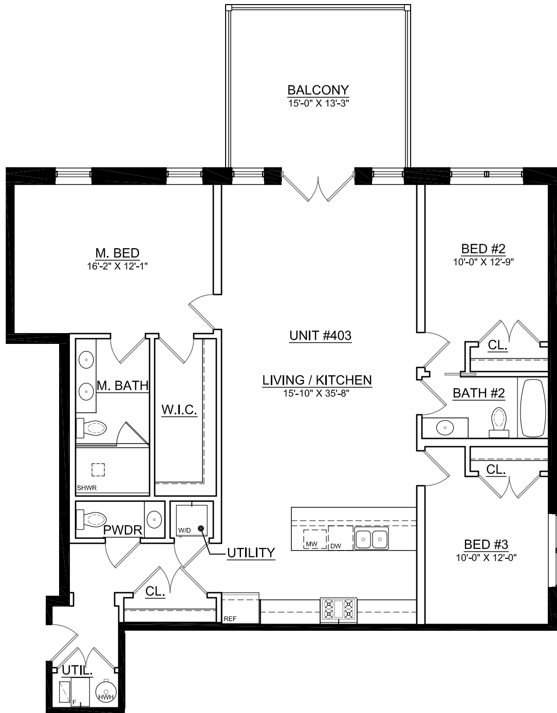
UNIT 403 SCALE: 1/8" = 1'-0"
